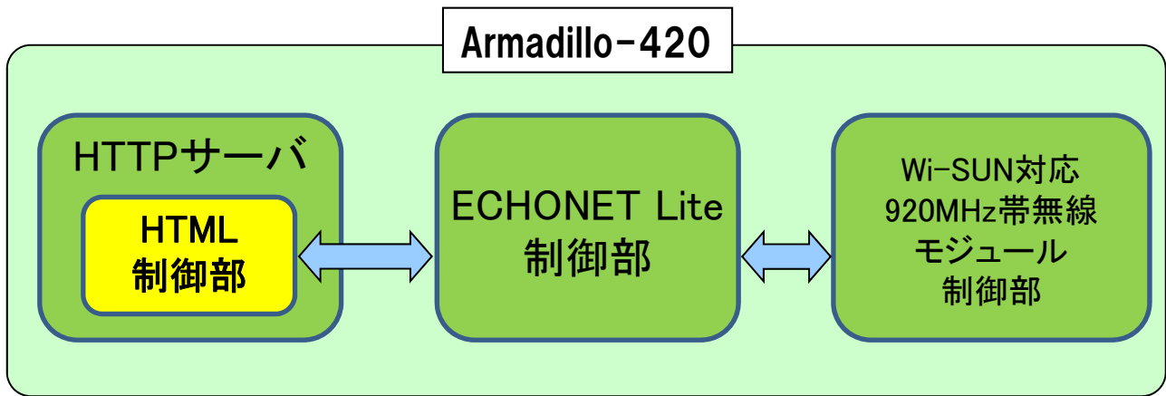
図1 コントローラ概略ブロック図
